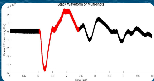
波形测试e-Boomer 550S @1000J
