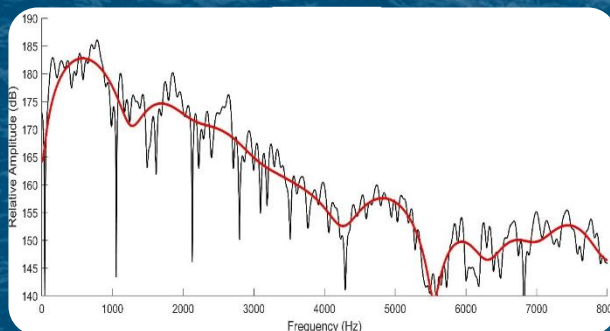
波形测试e-Boomer 550S @1000J
